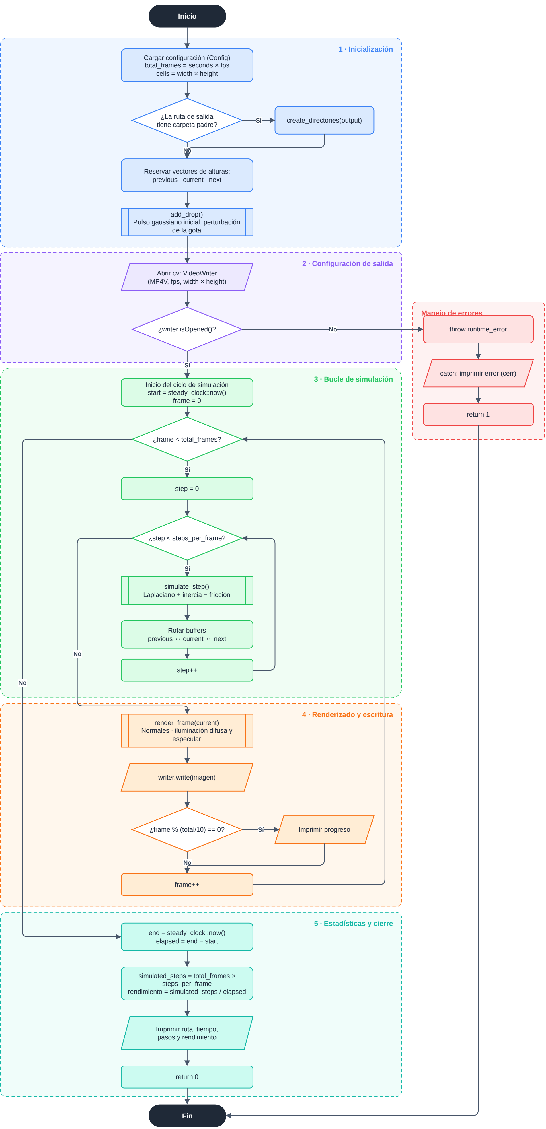
Diagrama de flujo — Simulación de gota (ecuación de onda 2D amortiguada)
